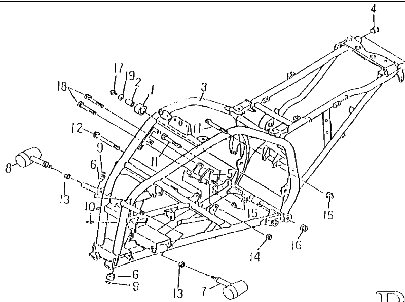
FIG.17 FRAME 車架
