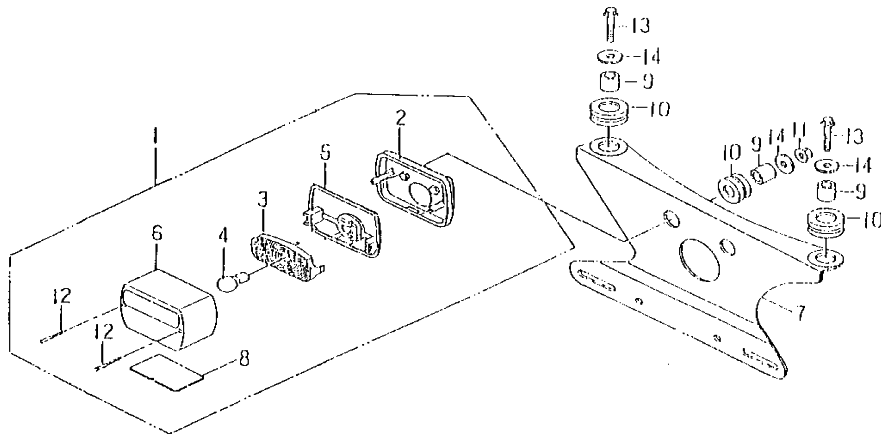
FIG.33 TAIL LIGHT 後燈
