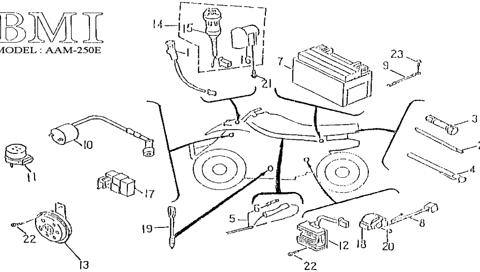
FIG.34 WIRE HARNESS 主電路配線
