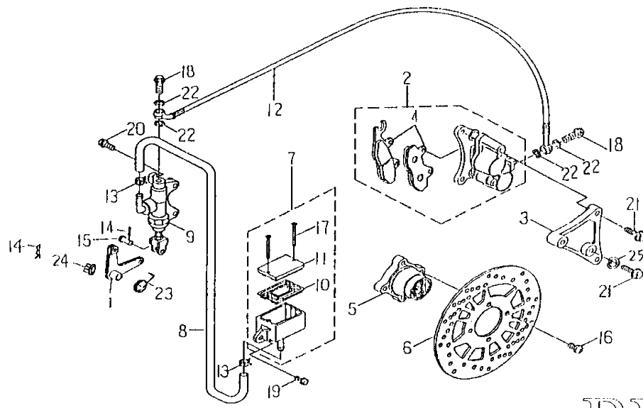
FIG.26 REAR BRAKE 後制車系統
