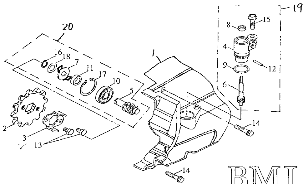
FIG.38 GEAR,SPEEDOMETER 速度表齒輪
