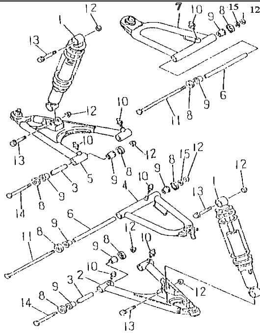
FIG.18 FRONT SUSPENSION 前懸吊系統
