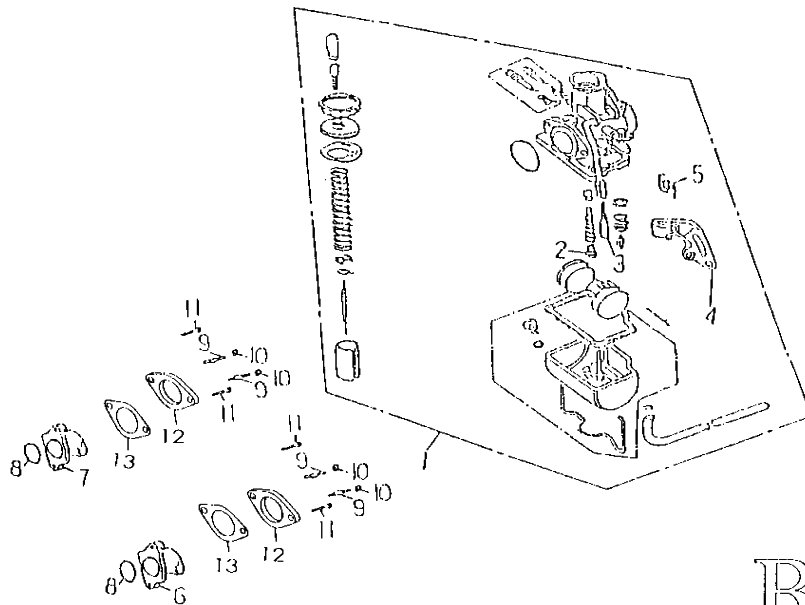
FIG.04 CARBURETOR 化油器
