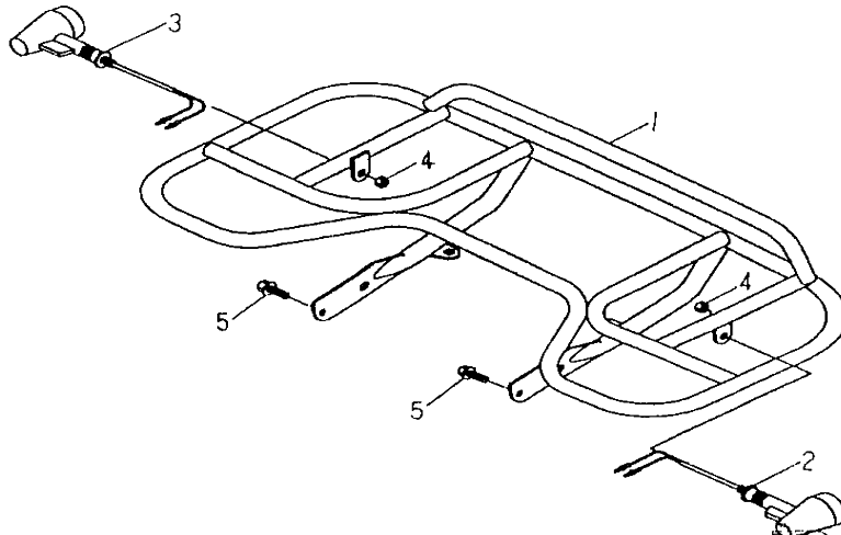
FIG.37 CARRIER,REAR 後架
