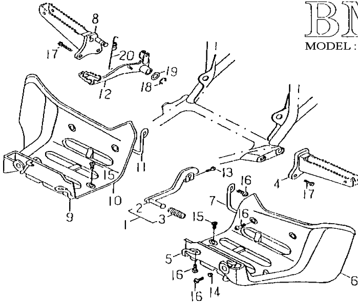
FIG.30 STAND FOOTREST 脚踏器
