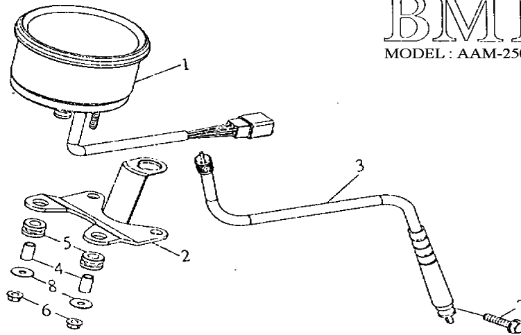
FIG.35 SPEEDOMETER 速度表
