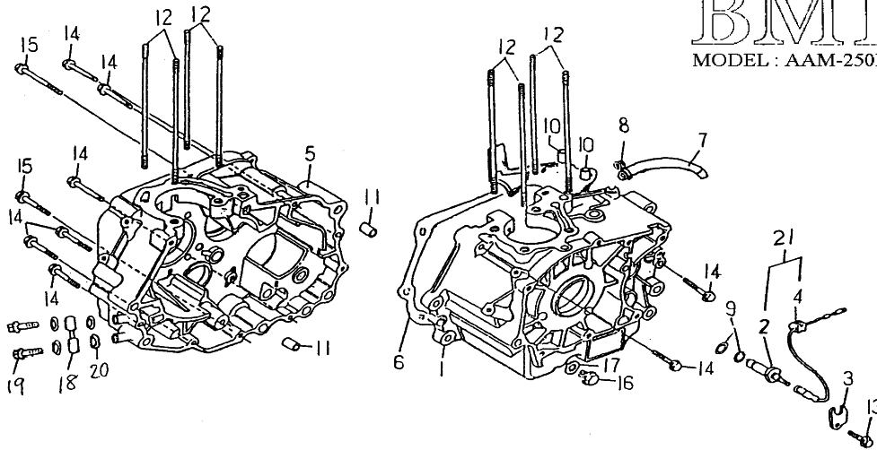
FIG.07 CRANKCASE 曲軸箱
